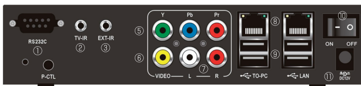
① RS232C：シリアルポート ② TV-IR：テレビリモートコントロール ③ EXT-IR：赤外線外部受光部 ④ P-CTL：リレイコントロール ⑤ コンポーネントビデオ出力 (Y-Pb-Pr / 最大 D4 出力) ⑥ コンポジットビデオ出力 ⑦ ステレオ音声出力 ⑧ イーサネットコネクタ × 2 ポート ⑨ USB 2.0 × 4 ポート ⑩ 電源スイッチ ⑪ 電源アダプタ差し込み口
